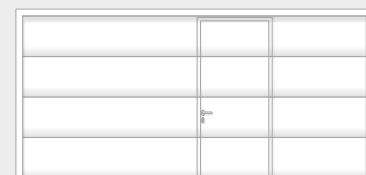
Disposición asimétrica para el ancho de la puerta BRB 3501 - 4250 mm - descentrado izquierda o derecha
