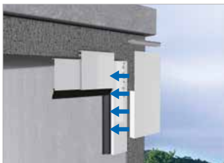
Solución universal, vista exterior
